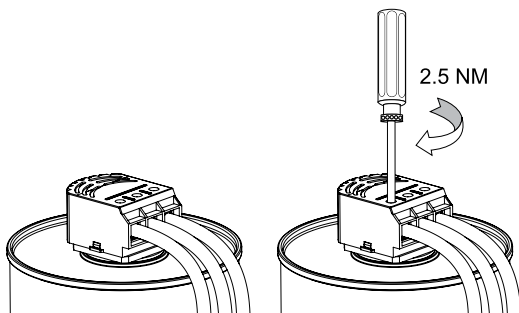
Stud Type
